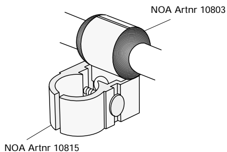
Horisontal infästning
