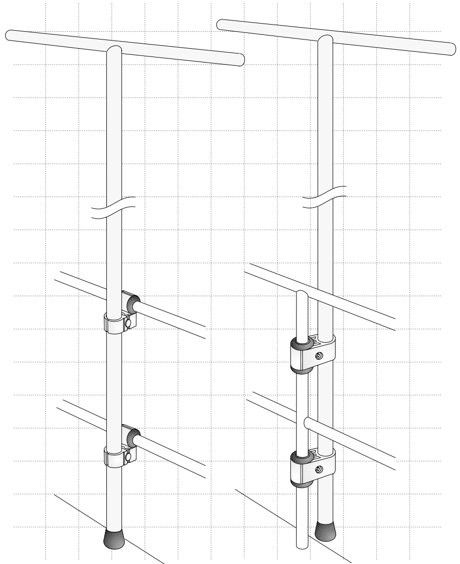
Horisontal infästning
